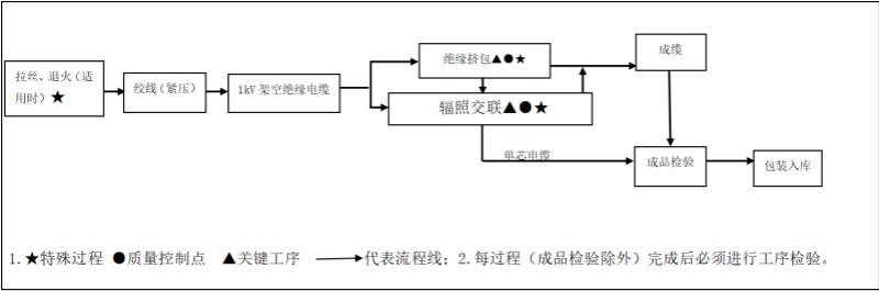
图 3-4 1kV 架空绝缘电缆工艺流程图
