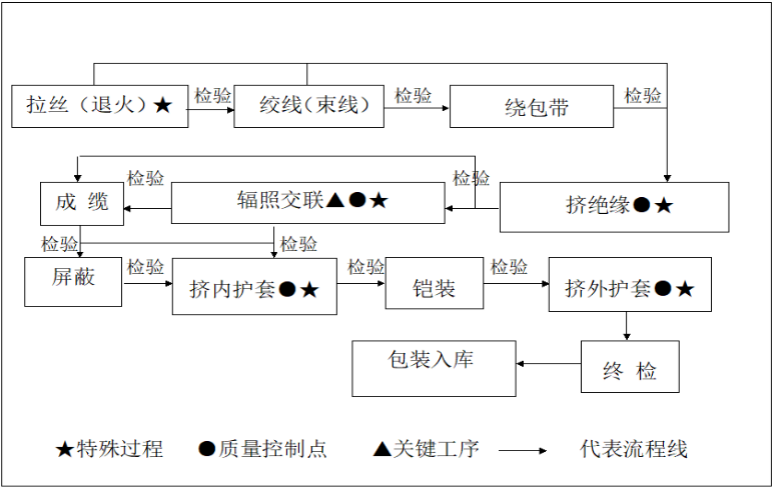
图 3-3 塑料绝缘控制电缆工艺流程图
